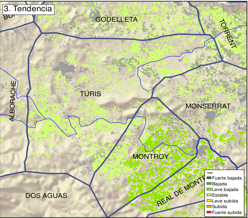
4. Densidad extratempranas
